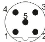
M12-B-codiert Stecker / Male M12 B-coded
