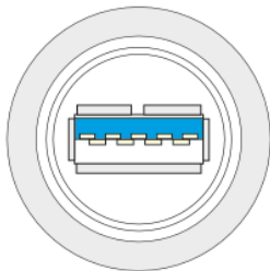
USB-A 3.0 Buchse / Female USB-A 3.0 22,5 mm Ausschnitt / 22,5 mm cutout
